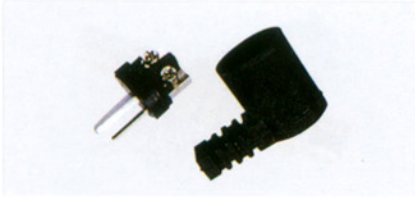
FC-A-0559 (0041) 2P DIN plug angle screw type
